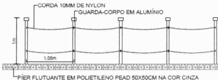
DETALHE GUARDA-CORPO
